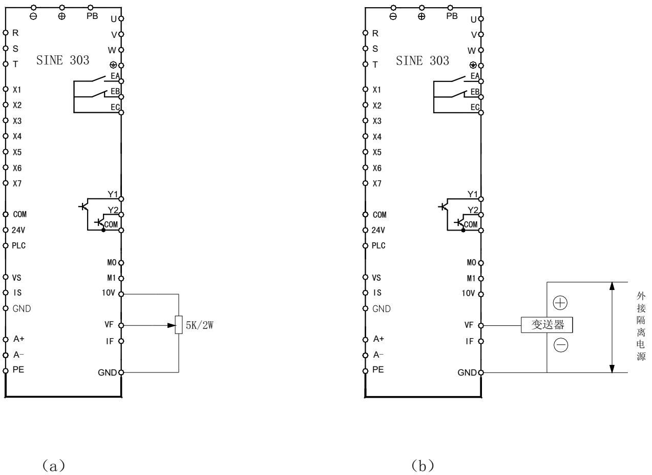
图 6-11 电压型反馈检测接线
