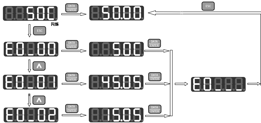
图 4-9 故障监视代码参数查询操作流程
