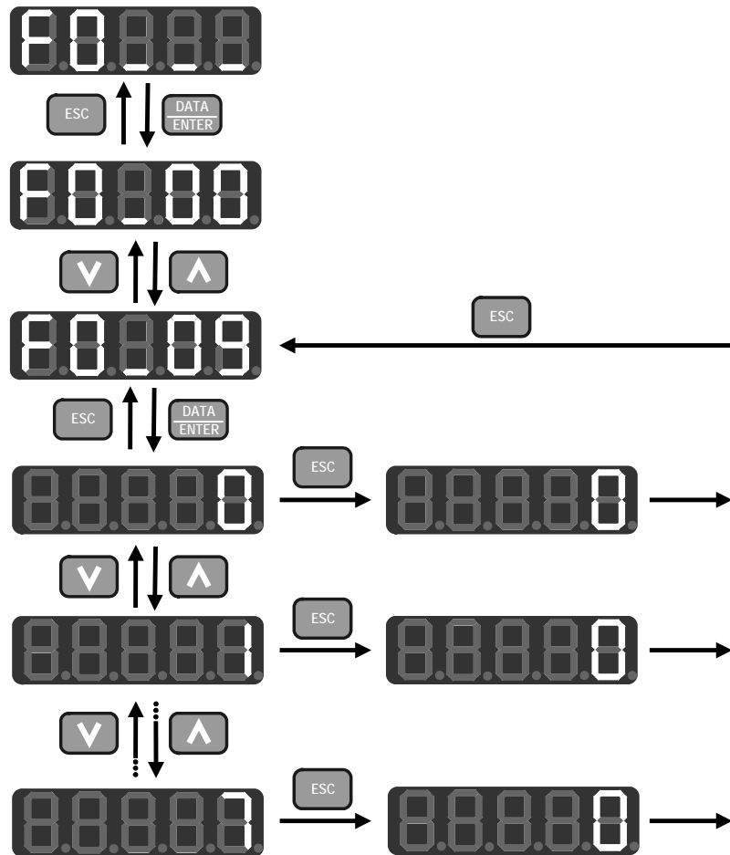
图 4-7 恢复修改前参数操作流程
