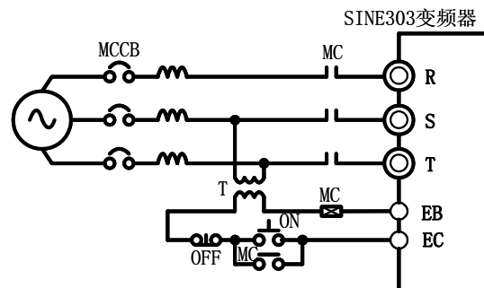
图 3-5 接入输入断路器
