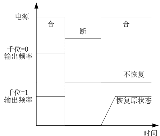
图 5-8 上电恢复示意图
