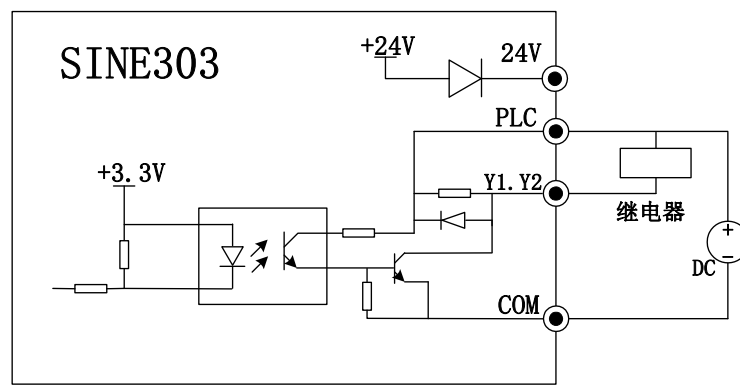
图 3-19 (b) 多功能输出端子用外部电源接线方式
