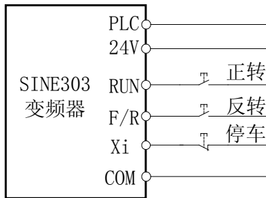
(a) F0.05=2 三线控制接线示意图
