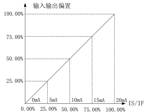
图 5-21 模拟电流输入 0~20mA
