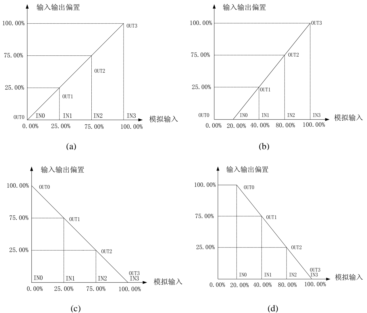
图 5-22 输入输出偏置
