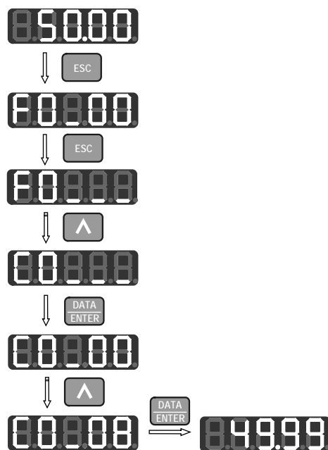
图 4-8 运行监视代码参数切换查询、修改操作流程
