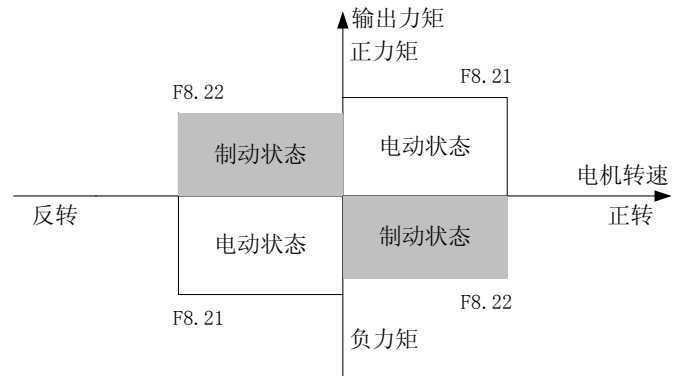
图 5-36 电制动力矩电流限定
