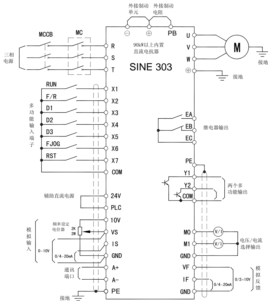
图 3-23 控制回路端子连接图
