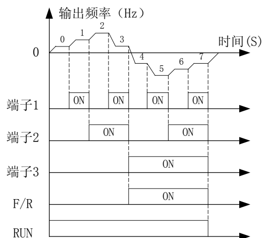
图 5-31 多段速度运行逻辑图
