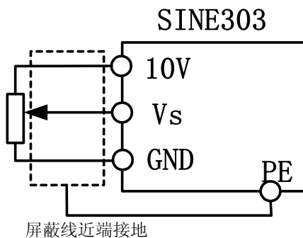
图 3-15(b) VS 端子配线图
