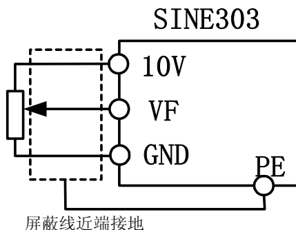
图 3-16 (b) VF 端子配线图
