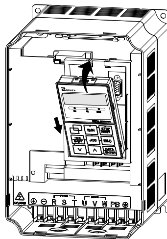
图 2-4 键盘安装图示
