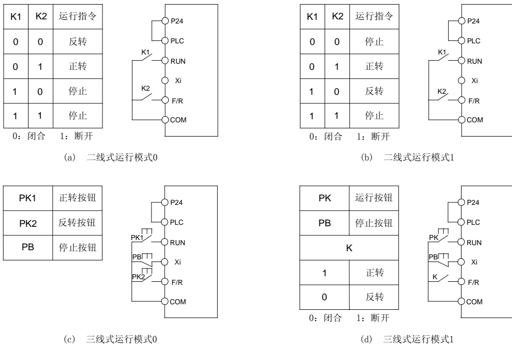
图 1-3 端子运行方式控制逻辑图
