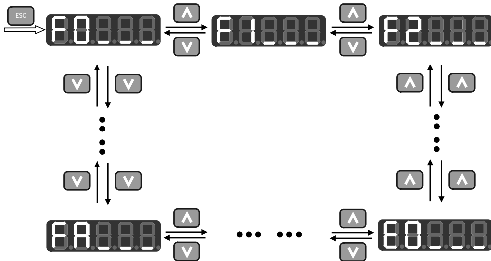
图 4-2 主菜单选择操作
