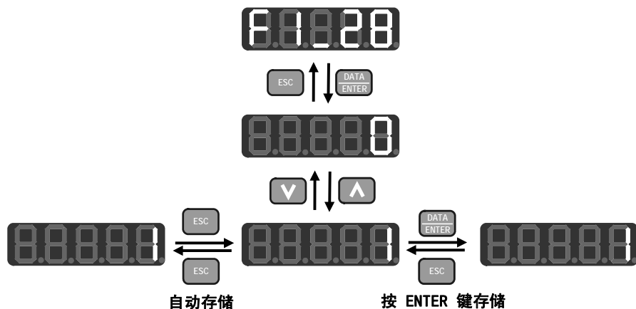
图 4-6 功能设定代码参数存储操作流程
