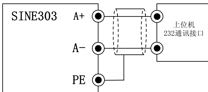
图 3-21 通讯端子配线
