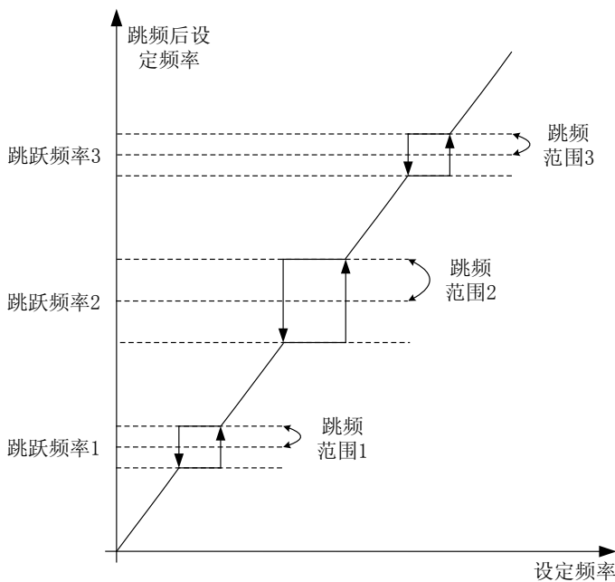
图 5-27 跳频
