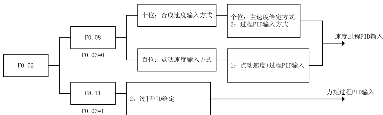
图 6-2 过程 PID 输入方式
