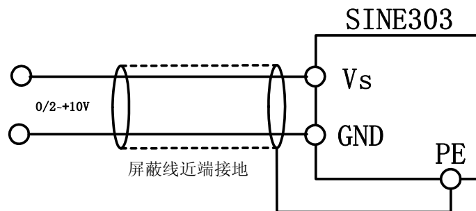
图 3-15(a) VS 端子配线图
