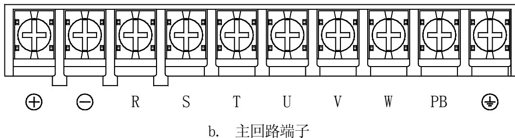
图 1-5 控制回路端子和主回路端子
