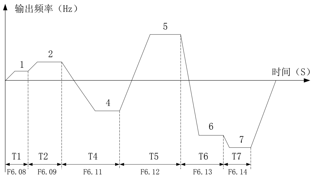
图 5-32 程序运行举例逻辑图
