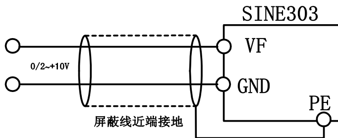
图 3-16 (a) VF 端子配线图
