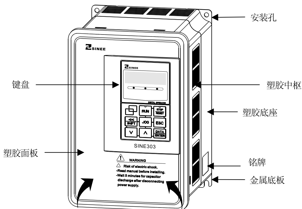
图 1-4 SINE303 系列变频器外型及部件
