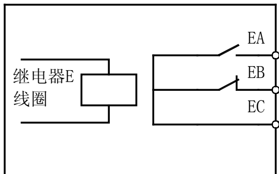
图 5-25 继电器触点
