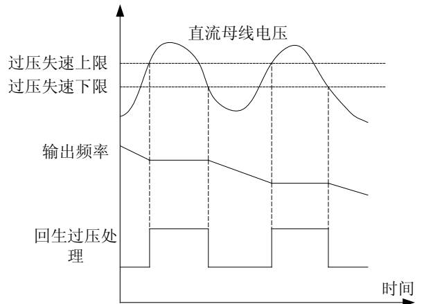
图 5-15 过压失速保护示意图
