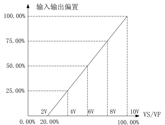
图 5-19 模拟电压输入 2~10V
