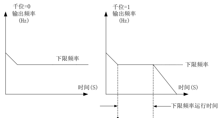
图 5-16 下限频率控制示意图
