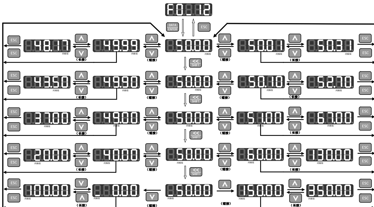
图 4-5 功能设定代码参数修改流程
