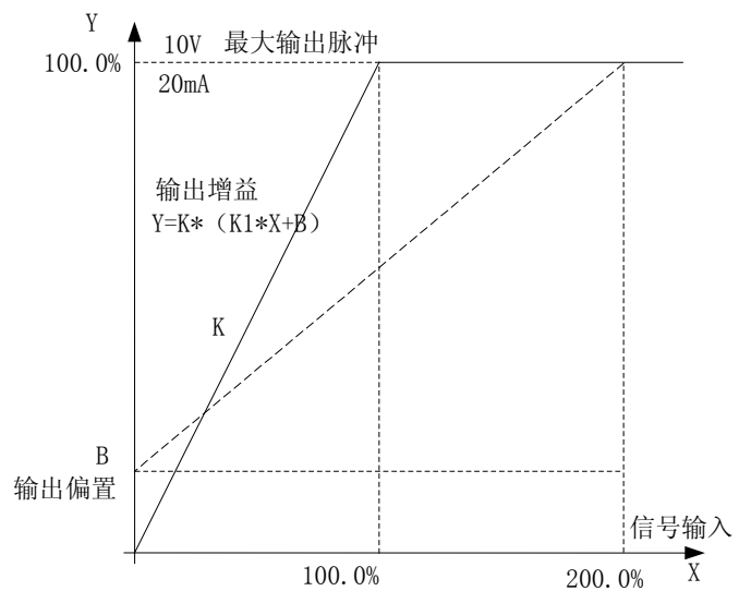
图 5—23 输出偏置曲线
