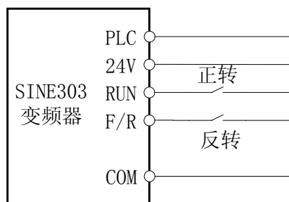
(c) F0.05=1 两线控制接线示意图
