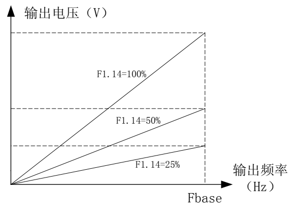
图 5-14 输出电压示意图
