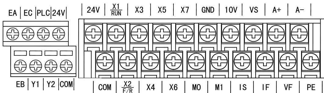
图 3-14 控制回路端子排列
