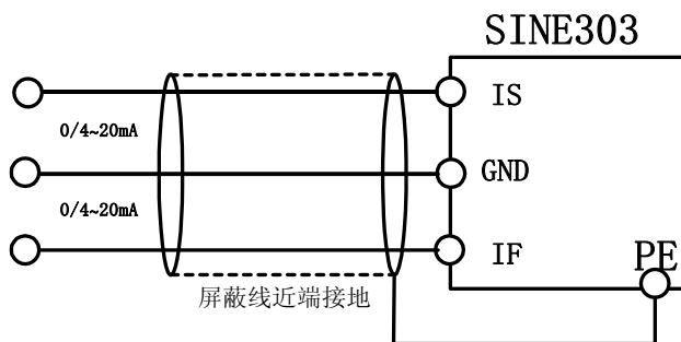
图 3-17 IS、IF 端子配线图
