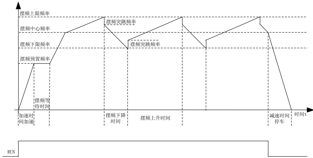
图 5—33 摆频运行逻辑图
