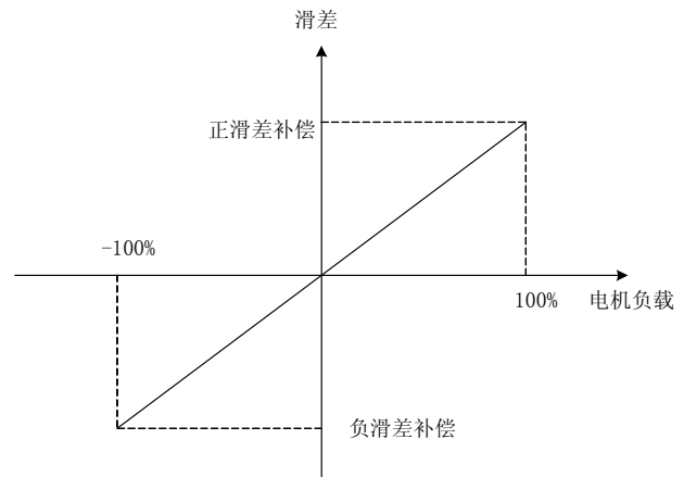
图 9-4 滑差补偿
