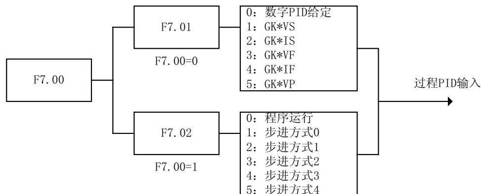
图 6-3 过程 PID 参考输入
