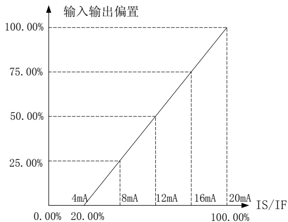
图 5-20 模拟电压输入 4~20mA
