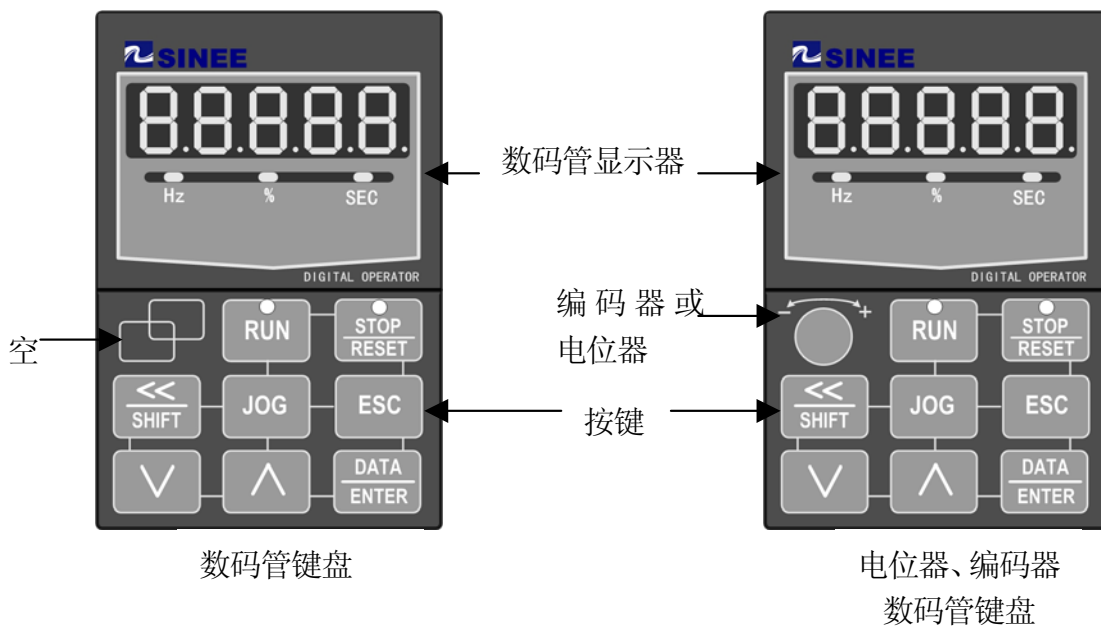
图 4-1 键盘各部件名称
