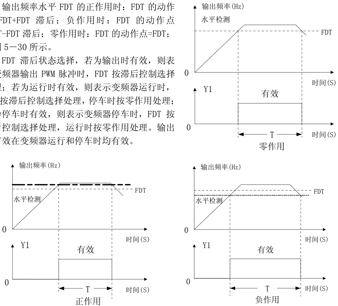
图 5-30 输出频率水平 FDT
