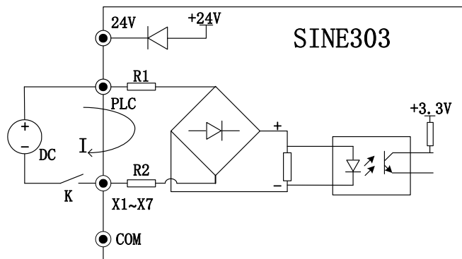
图 3-18 (b) 使用外部电源的连接方式
