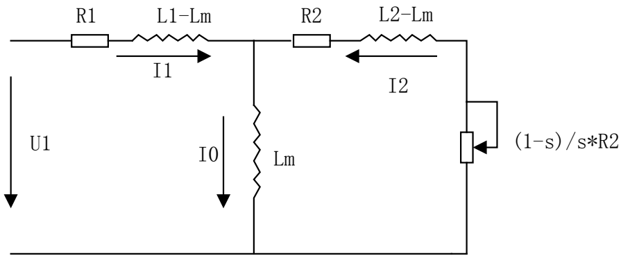
图 5—37 异步电动机稳态等效模型
