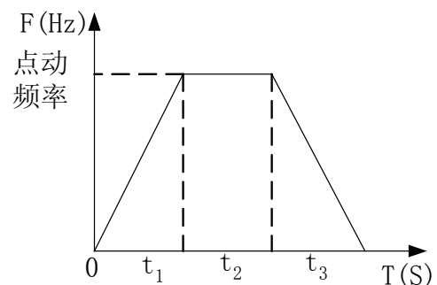
图 5-4 点动运行参数示意图
