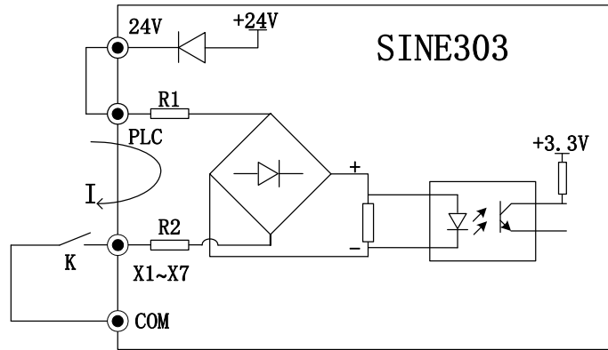
图 3-18 (a) 使用内部 24V 电源的连接方式
