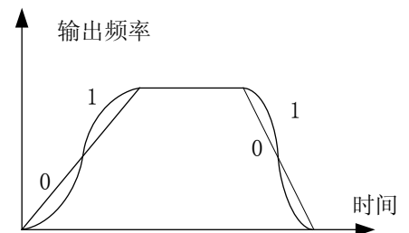
图 5-9 加速/减速模式
