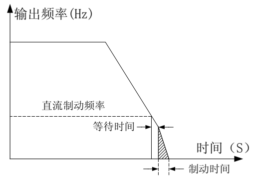
图 5-11 停车减速直流制动过程
