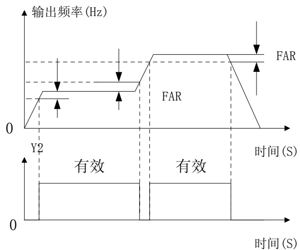
图 5-29 输出频率范围 FAR
