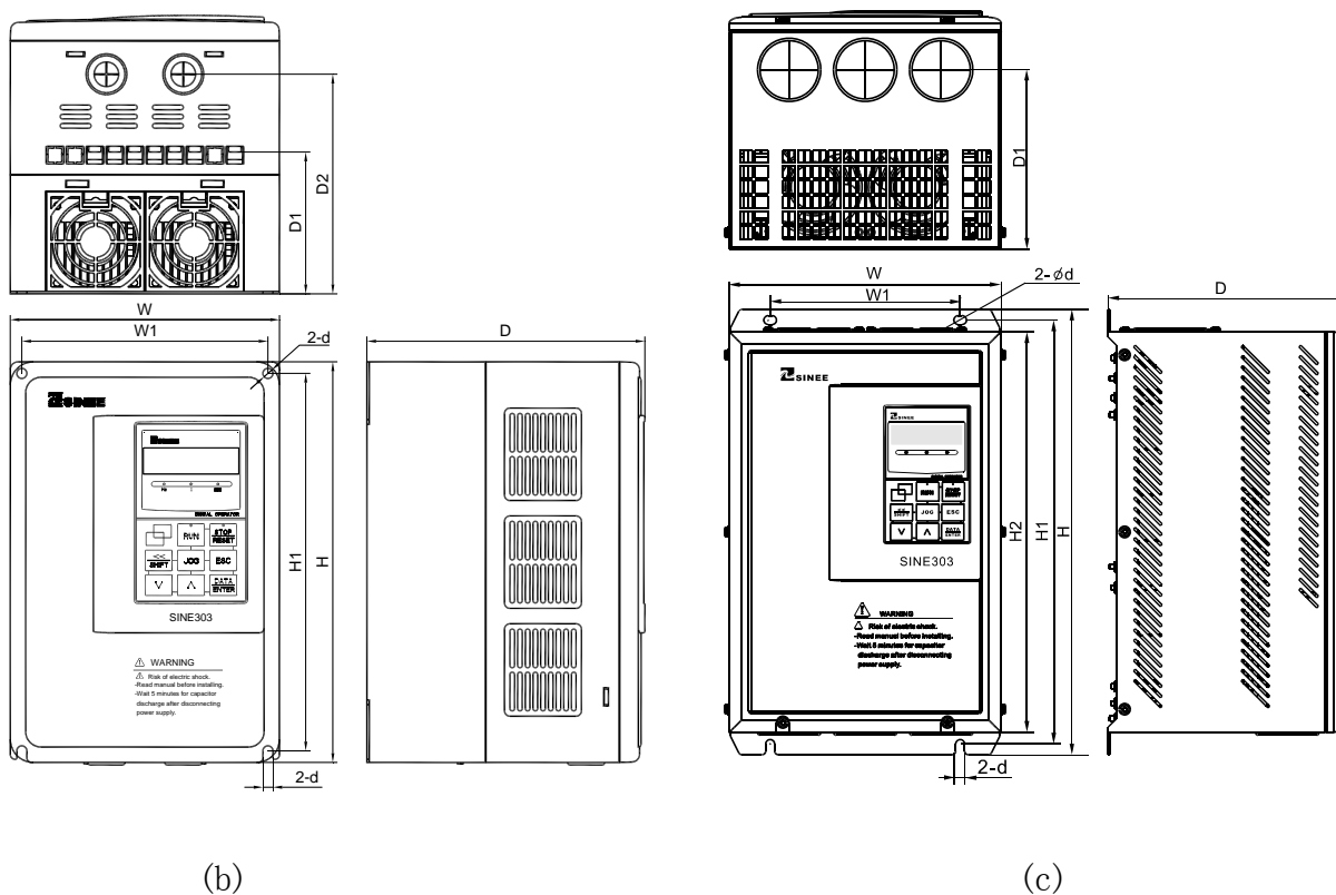
图 2-1 SINE303 系列开环矢量控制变频器和键盘外形尺寸图
