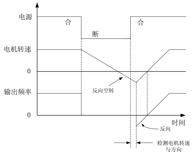
图 5-7 转速追踪再启动示意图
