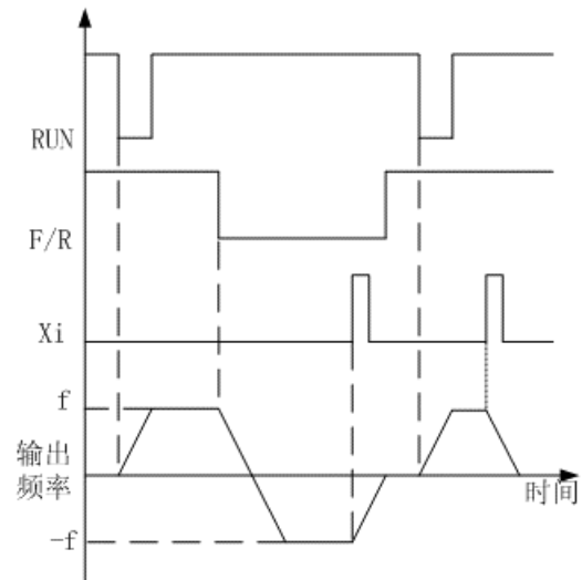
(d) F1.01=X0, F0.05=3 运行正/反转逻辑 图 5-3 三线控制
