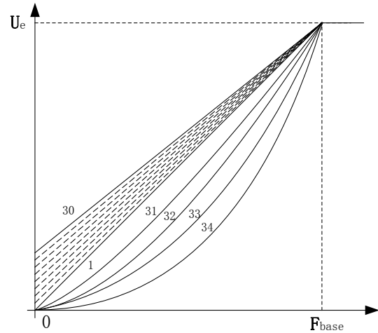
图 5-6 固定转矩提升曲线
