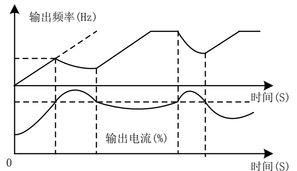
图 5-12 电流限幅动作过程
