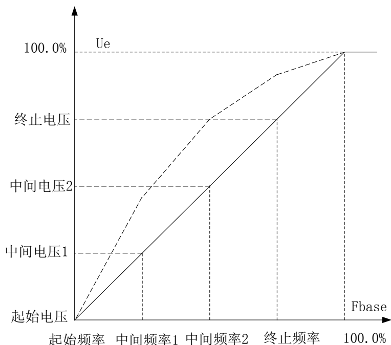
图 5-28 V/F 曲线设定
