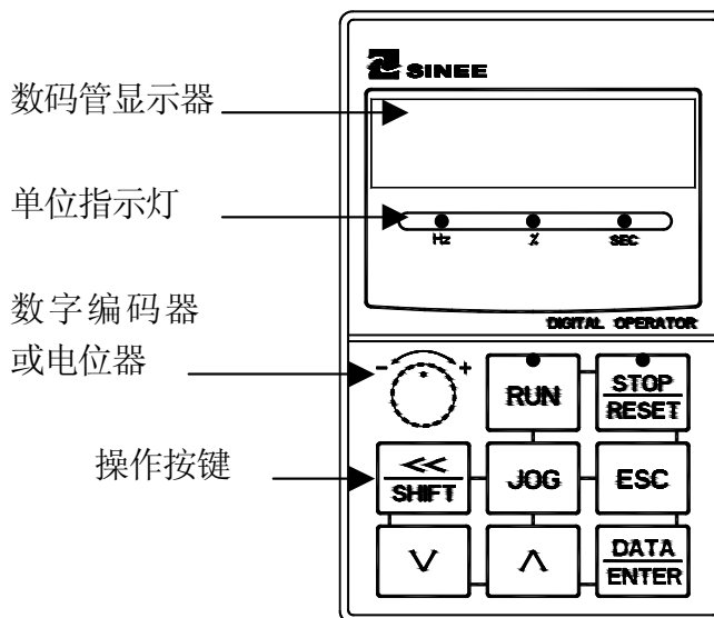
图 1-6 键盘图示
