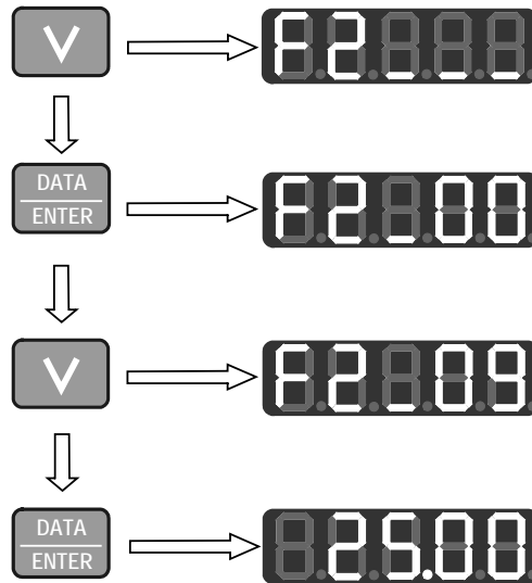
图 4-4 功能设定代码参数查询操作流程
