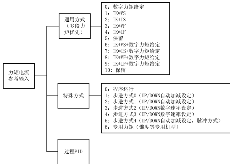
图 1-2 力矩输入方式示意图
