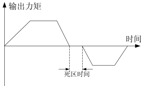
图 5-35 正/负力矩死区时间
