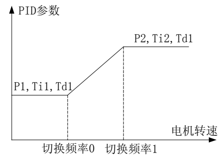
图 5-34 PID 参数示意图
