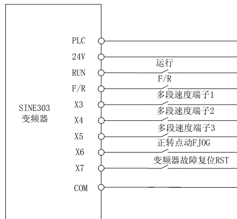
图 5-1 端子控制接线示意图
