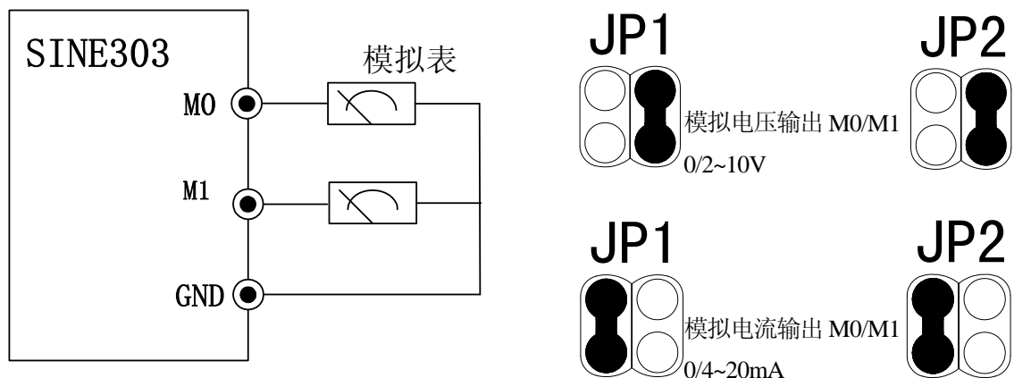
图 3-20 模拟输出端子配线
