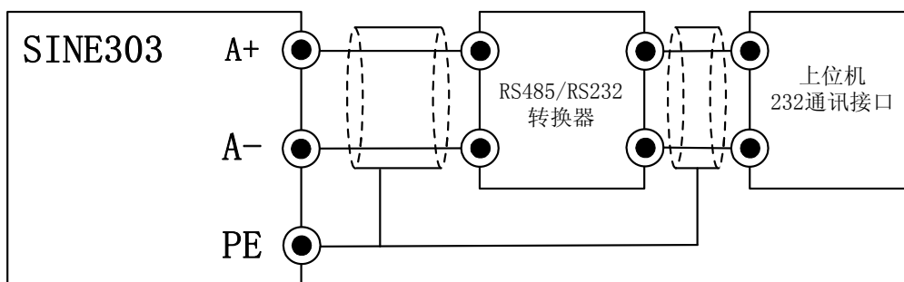
图 3-22 通讯端子配线
